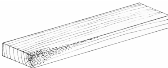
Gambar 12 - Cara mengukur dan menilai cacat lapuk
