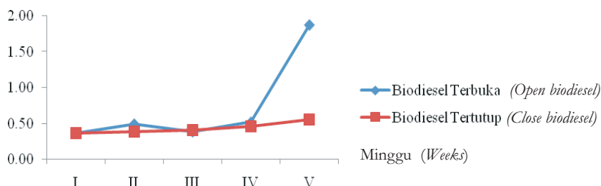
Gambar 3. Perubahan bilangan asam biodiesel pada kondisi berbeda Figure 3. Change of biodiesel acid values at different conditions
